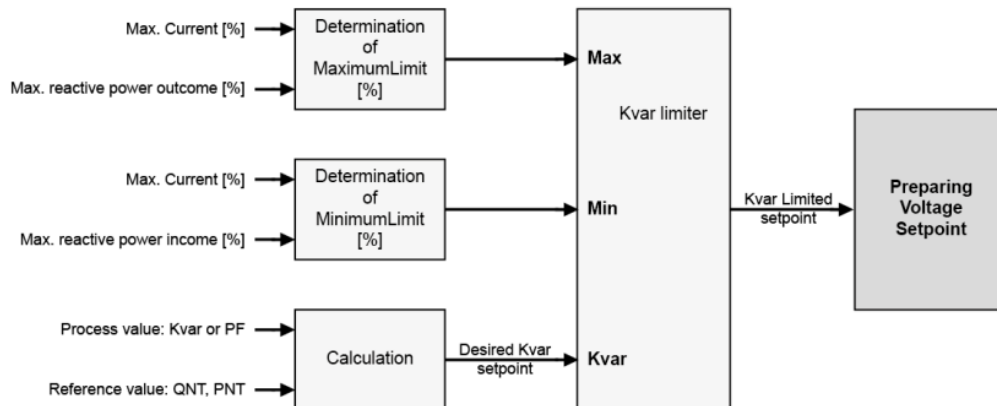
Abb. 176: Der kvar-Sollwert wird beschränkt, um den Generator zu schützen.
